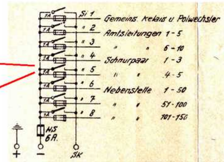
Auszug aus Schaltung S2e-21/8 II
