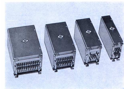
BILD 4 FSK-Relais zum Einbau in Relaischienen
