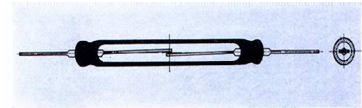
BILD 1 Clare-Reedkontakt
