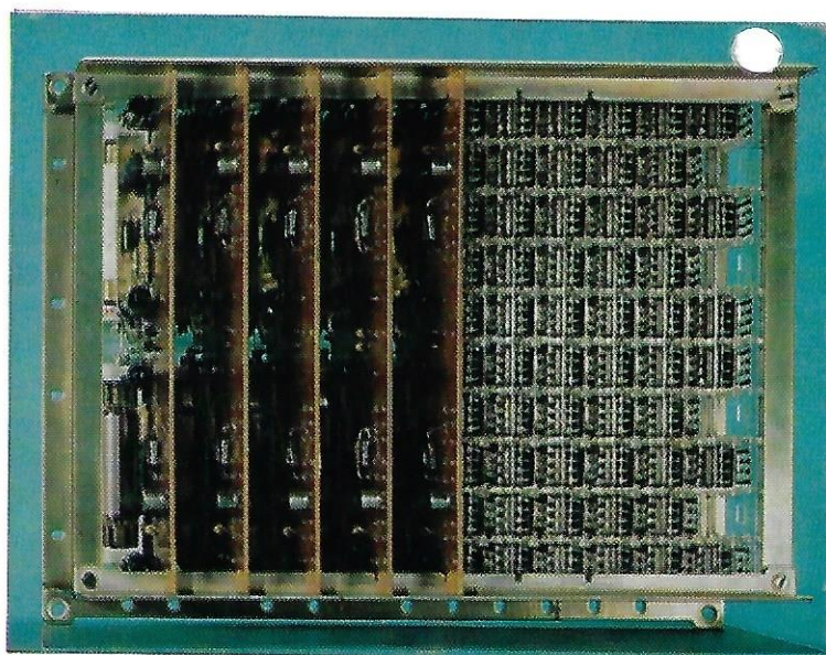
B I L D 6 Baugruppe, bestehend aus dem Koppelvielfach der Koppelstufe A sowie den Anschlußorganen und Steuerrelais für 10 Nebenstellen
