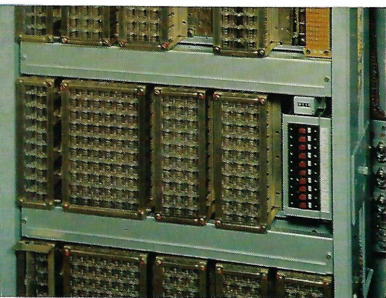
B I L D 5 Ausschnitt aus der Koppelstufe C
