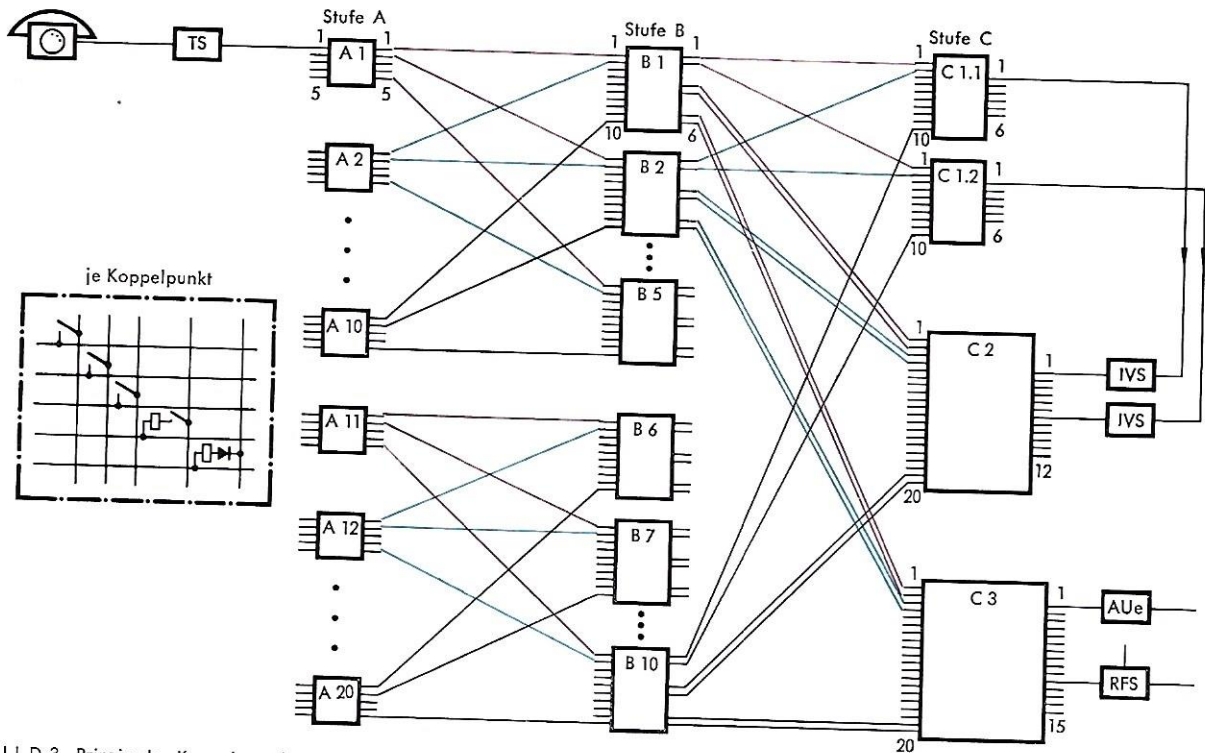
BILD 3 Prinzip der Koppelanordnung
