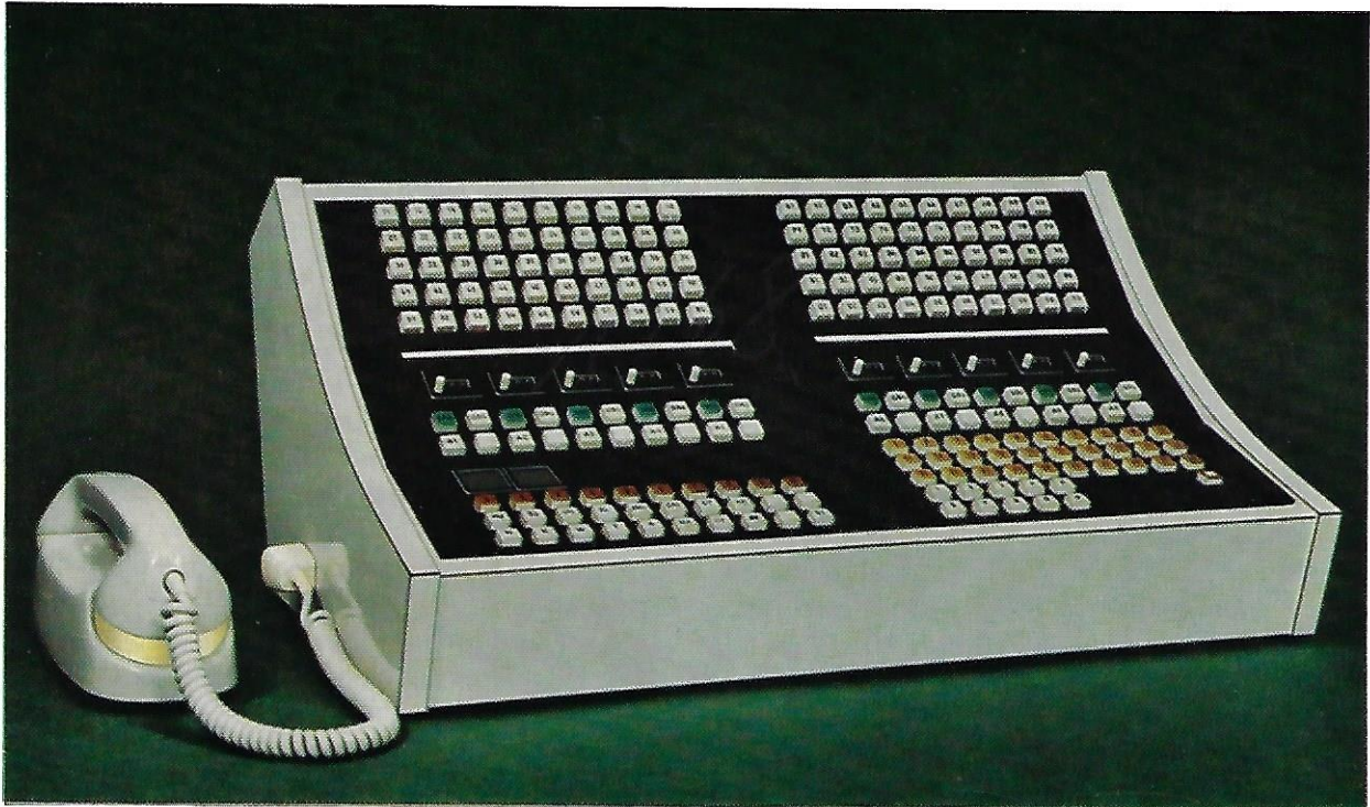
B I L D 2 Vermittlungsapparat für die TN-Nebenstellenzentrale der Baustufe II G in Multireed-Technik
