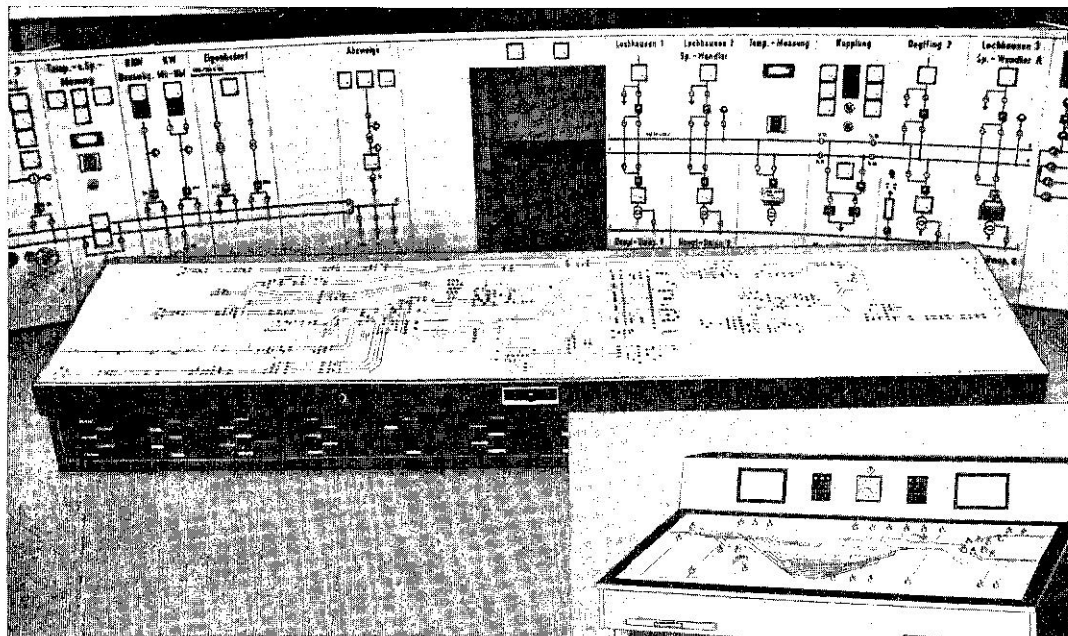
Fernkommandopulte für den elektrifizierten Bahnbetrieb
