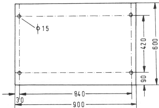
Boden-Befestigungsmaße
