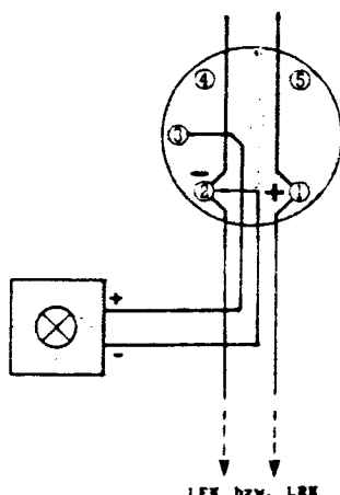
Anschluß einer externen Anzeige
