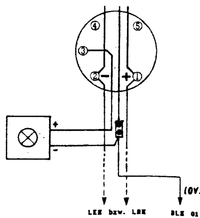
Anschluß einer externen Anzeige (zus. 0V-Leitung)
