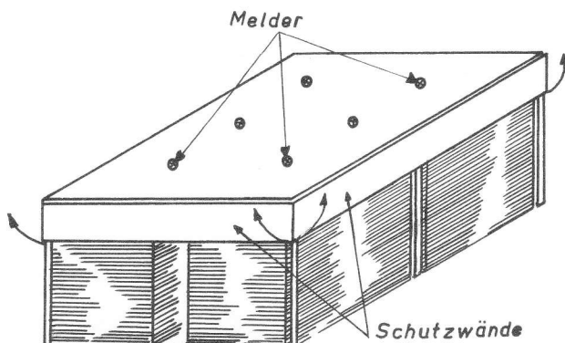
Offene Halle mit Flachdach. Wenn das Lagergut bis dicht unter das Dach gestapelt wird, empfiehlt sich die Anbringung von aufklappbaren Schutzwänden.
