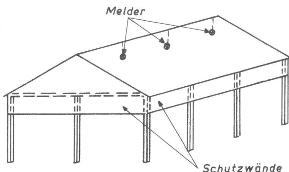
Offene Halle mit Giebeldach
