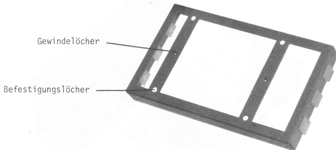
Bild 2 Aufputzrahmen
