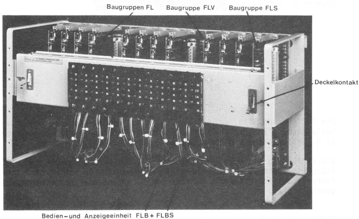
Bedien- und Anzeigeeinheit FLB + FLBS
