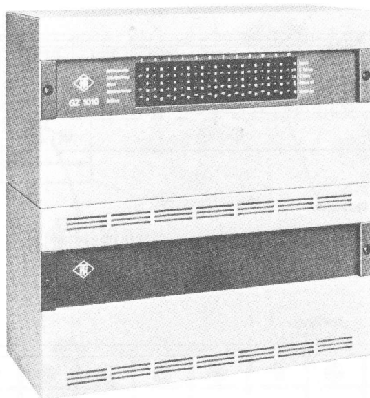
Gefahrenmeldezentrale GZ 1010 mit Zusatzgehäuse für die Energieversorgung
