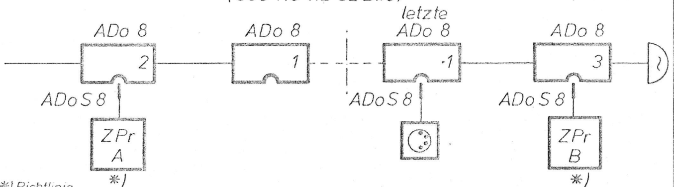
ZPr A und ZPr B an tragbare FeAp 613-616 (386 110 112 Sz Bl. 9)
