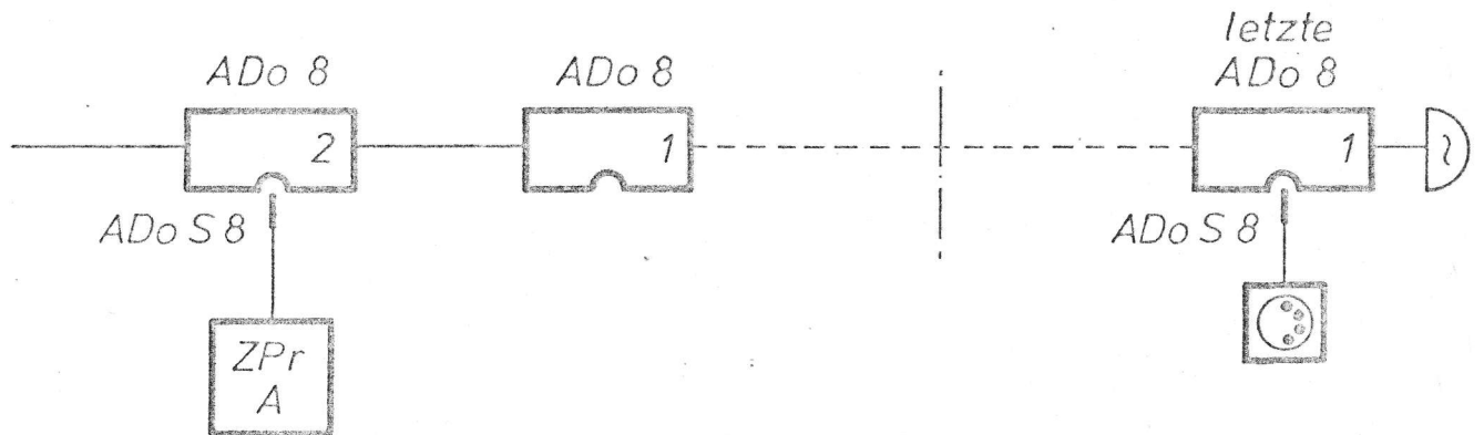
ZPr A an tragbare FeAp 613-616 (386 110 112 Sz Bl. 7)
