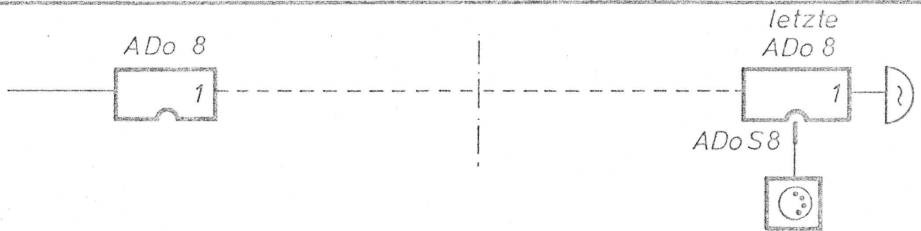
Anschlußdosenanlage 8-polig für FeAp 613-616 (386 110 112 Sz Bl. 6)
