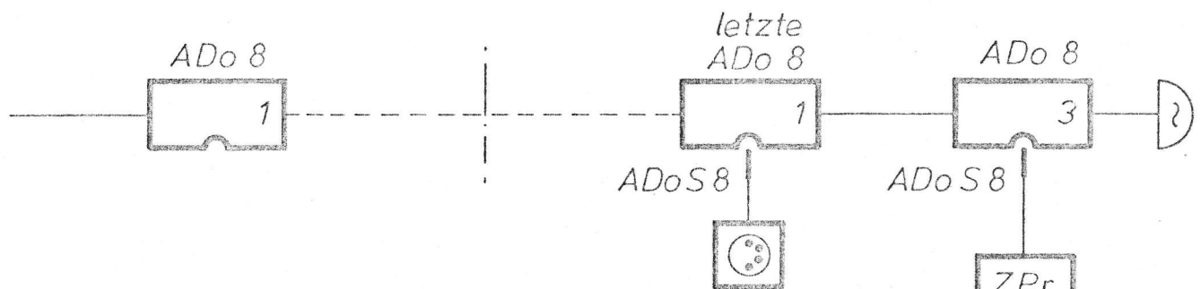
ZPr B an tragbare FeAp 613-616 (386 110 112 Sz Bl. 8)
