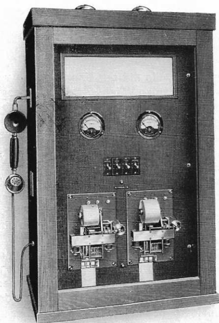
F 275 M Feuermeldezentrale „Duplex“ „System 2“
