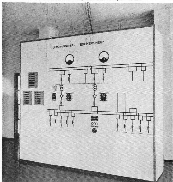
Fernkommandotafel in einer Schaltwarte
