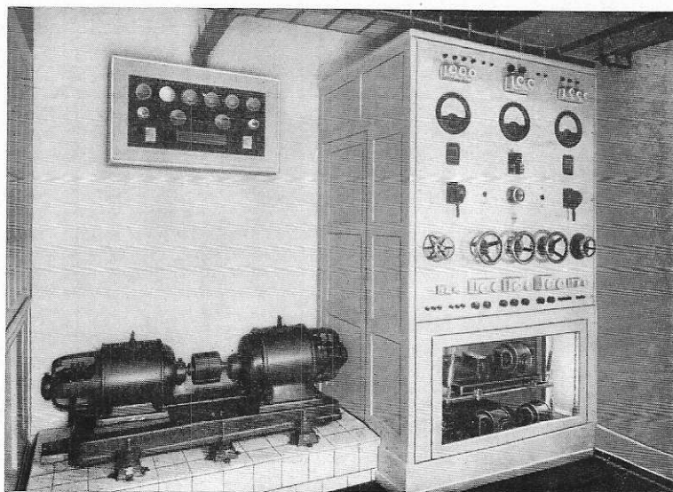
Schalttafel, Überwachungstafel, Lade- und Signalmaschinen der Fernsprechanlage im Rathaus Kassel.
