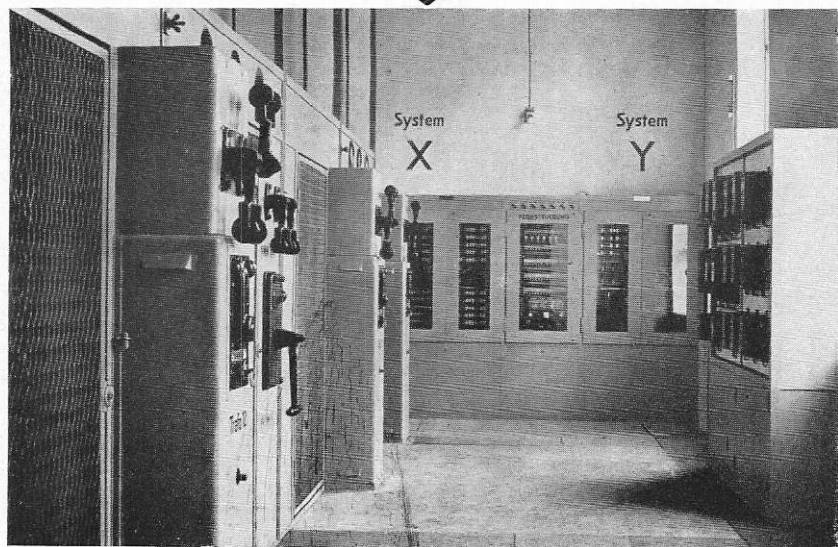
Teilansicht eines ferngesteuerten Umspannwerkes
