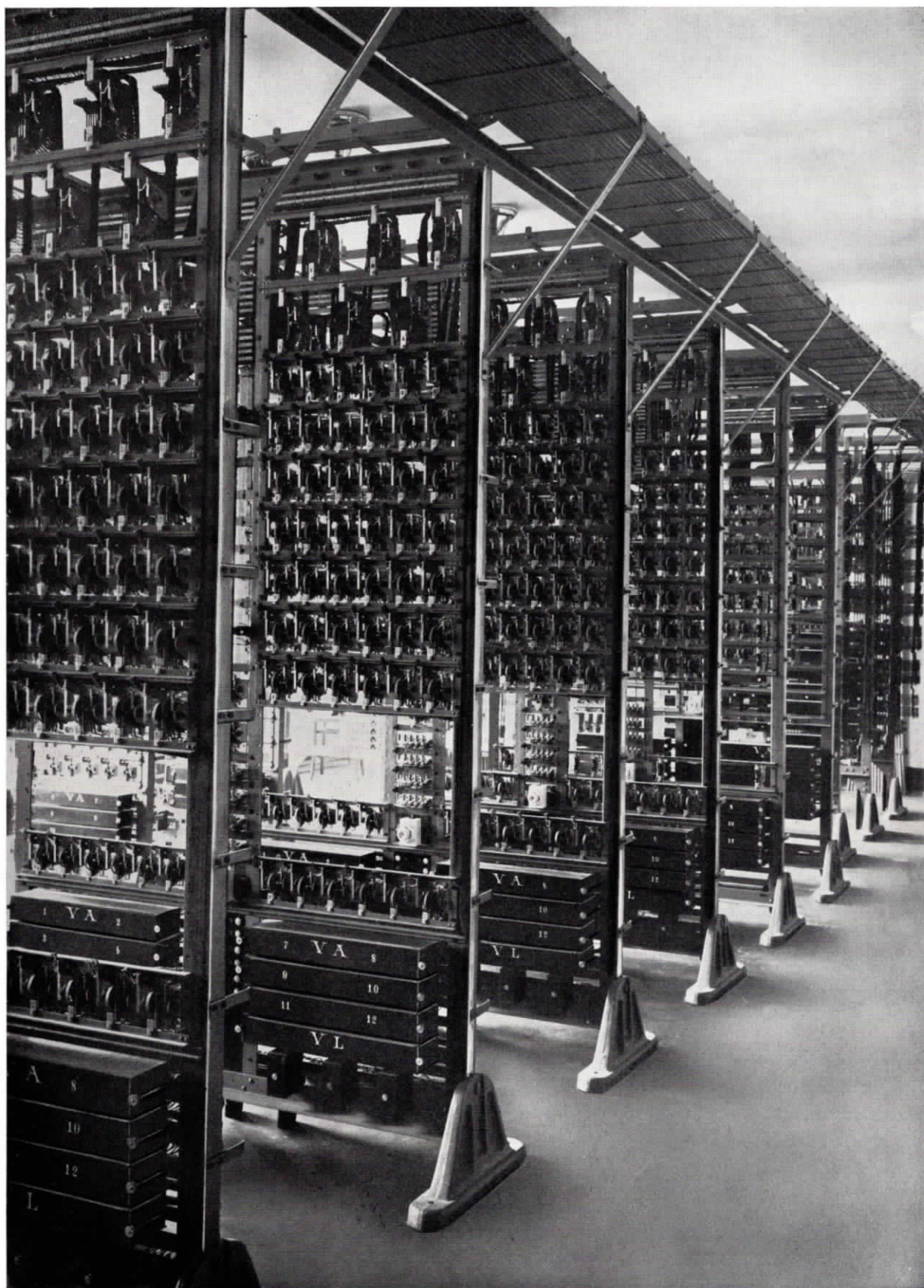
Abb. 5. SA-Fernsprechzentrale, Skodawerke Prag
