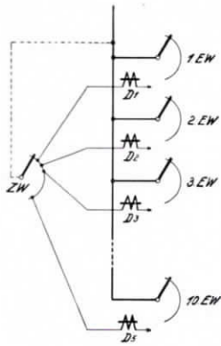
Abb. 11. 100-teiliger LW (Defa- ditisches Drehwählersystem)
