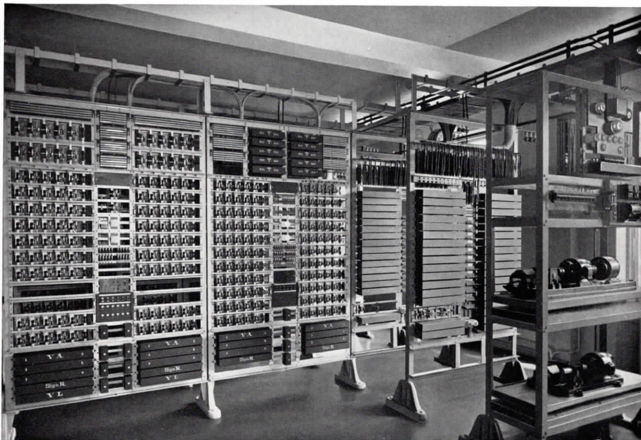
Abb. 6. SA-fernsprechanlage, Städt. Krankenhaus Frankfurt a. M.
