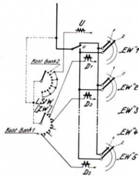
Abb. 12. 280-teiliger LW (Raststellensystem)
