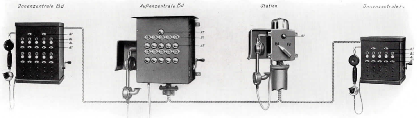
Abb. 25. Rangiertelefonanlage, Ausführung Hauptbahnhof Frankfurt a. M.
