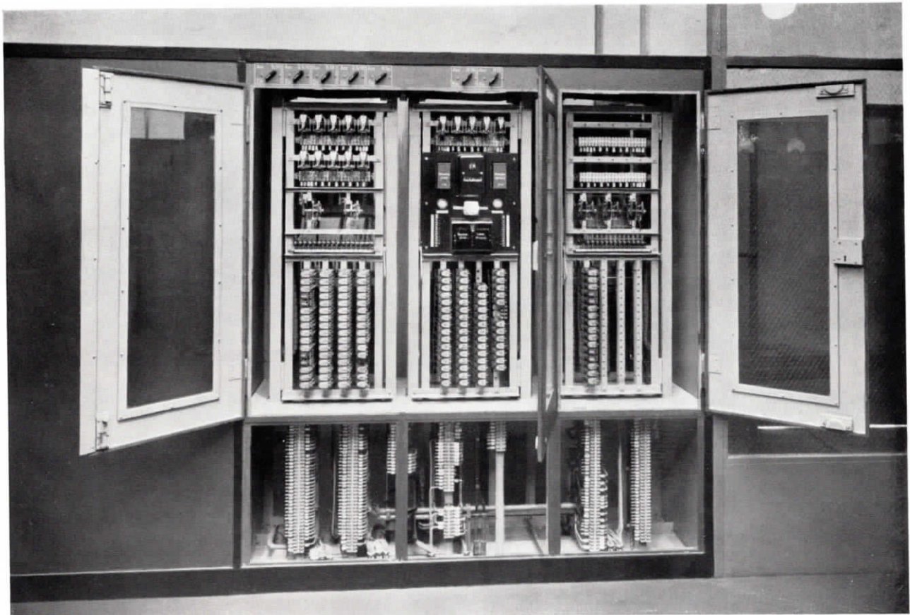
Abb. 34. Kommandoübertragereinrichtung in einer bedienungslosen Unterstation
