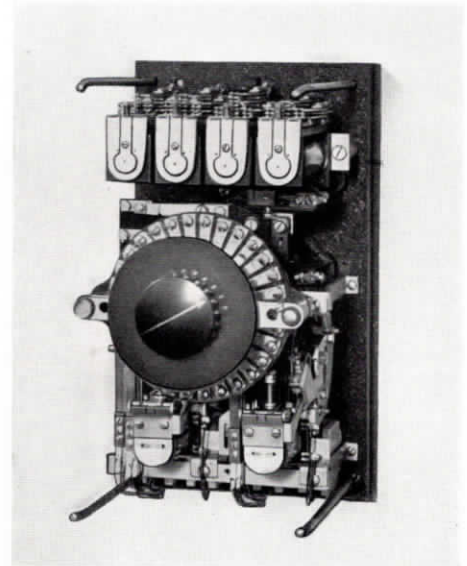
Abb. 37. Zeitstafelschaltwerk, Schutzklappe abgenommen
