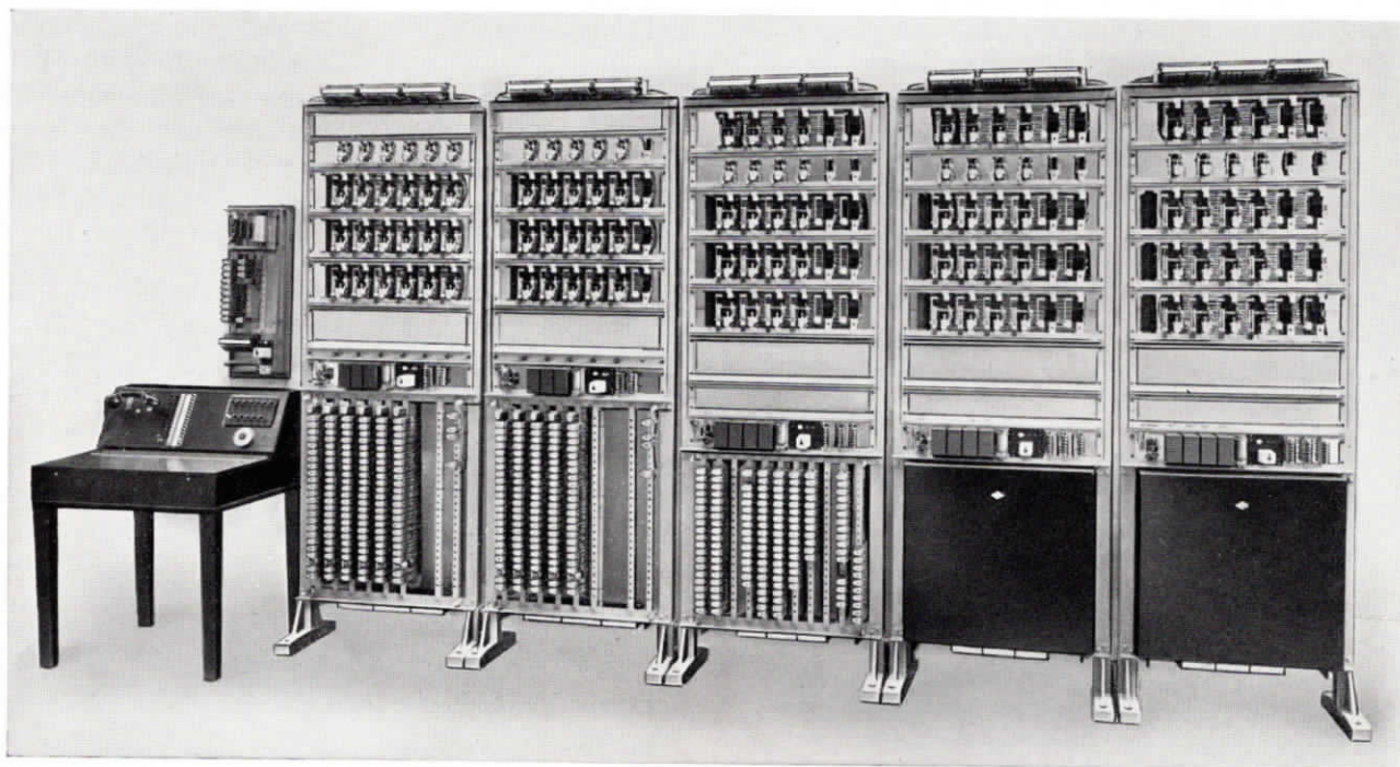
Abb. 15. Mittlere SA-Nebenstellenanlage 2 in reichspostmäßiger Ausführung. Relaischuhklappen teilweise abgenommen.
