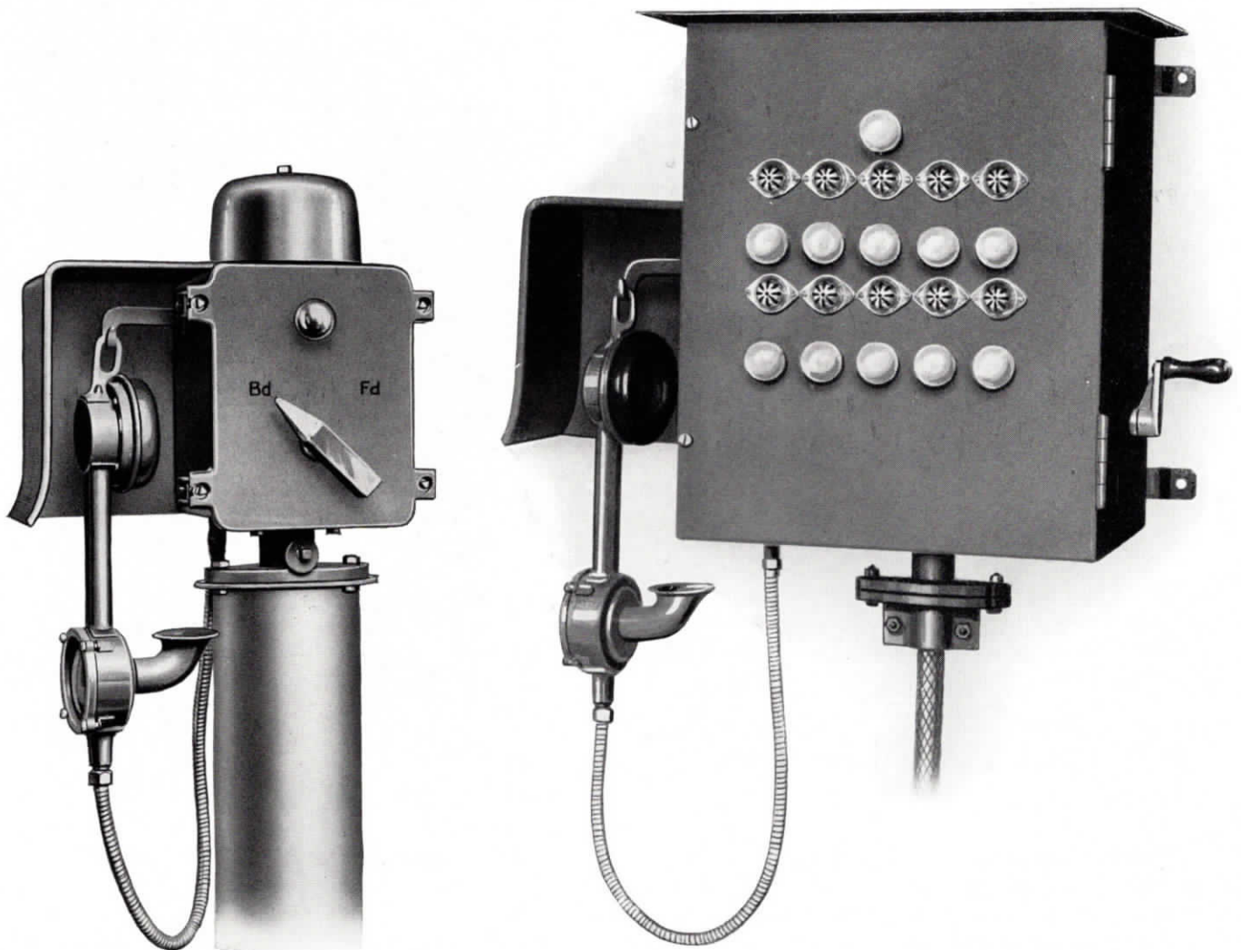
Abb. 27. Vermittlungszentrale in wetterfester Ausführung für Rangierfernprechanlagen
