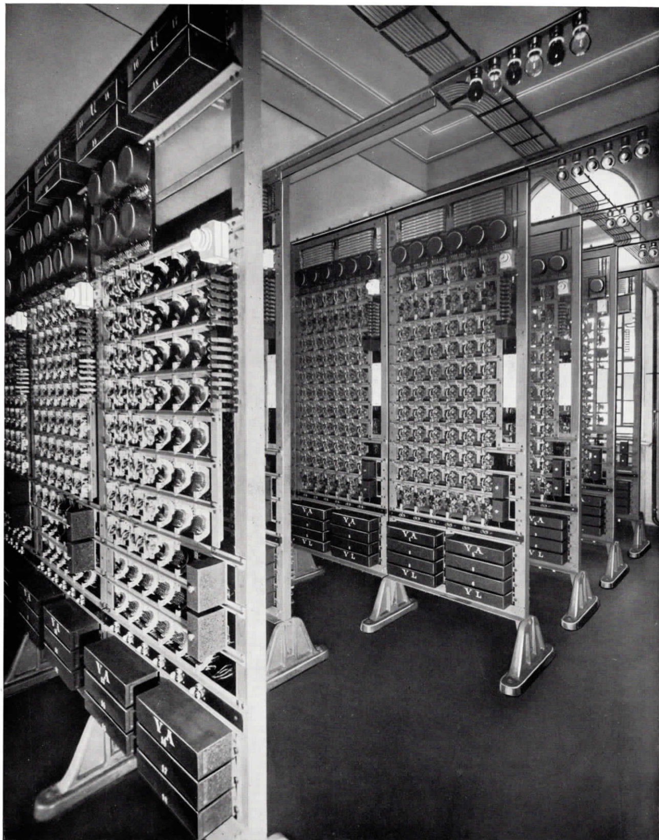
Abb. 3. Fernsprech-Hauptzentrale, Polizeipräsidium Berlin
