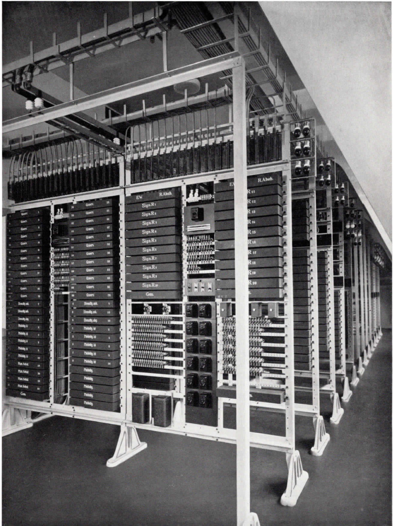
Abb. 7. Halbautomatische Nebenstellenanlage, Stadtverwaltung Frankfurt a. M. (vergl. Abb. 21)
