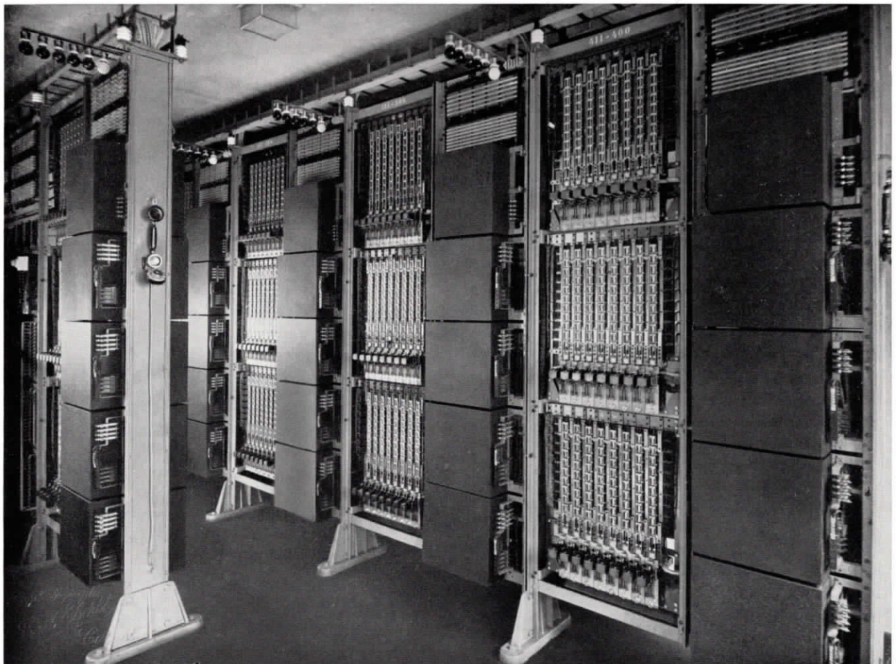
Abb. 17. SA-Bernsprechzentrale (Stangenwählersystem) im Rathaus Kassel
