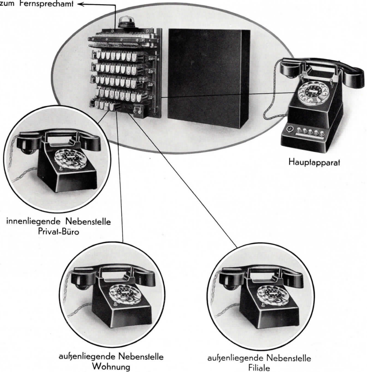
Abb. 20. SA-Nebenstellen-Kleinanlage (Type Reford)
