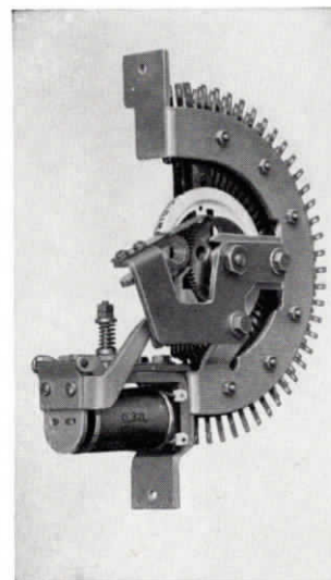
Abb. 9. 30 teiliger Drehwähler
