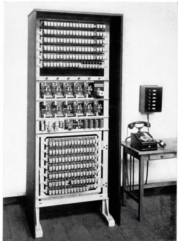
Abb. 14. Vordere Schutzwand abgenommen
