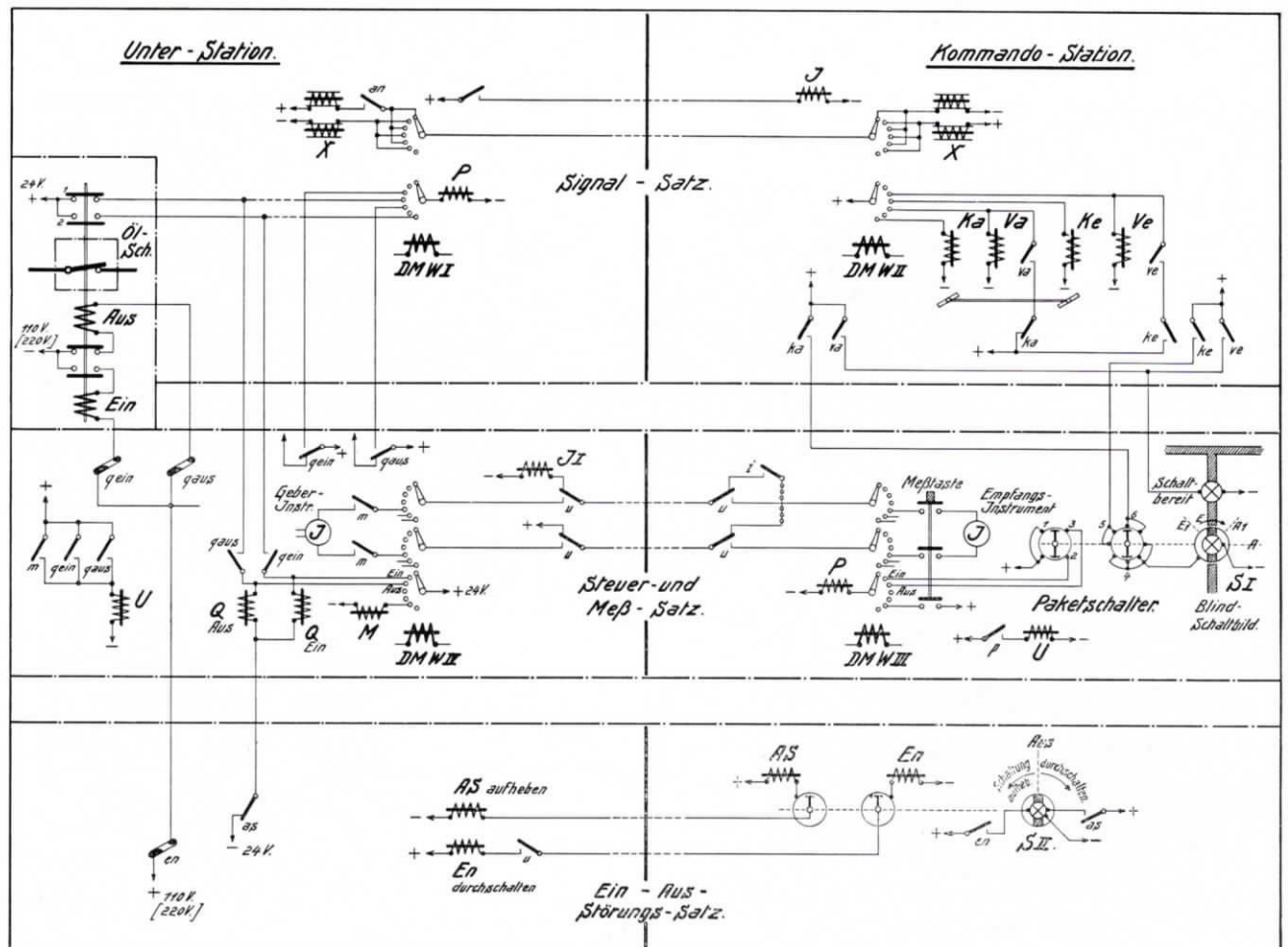
Abb. 32. Fernsteueranlage (Prinzipialschaltbild)
