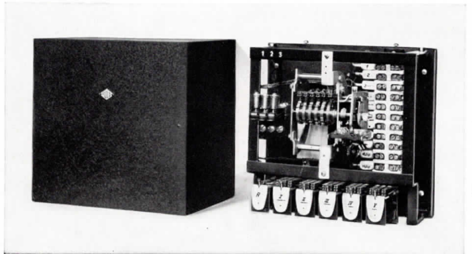
Abb. 30. Steuerstelle für selbsttätige, akustische Morseignale
