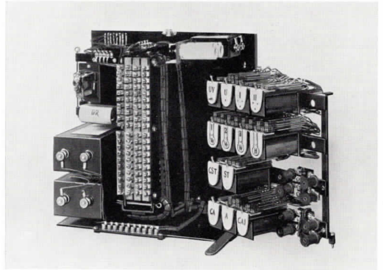
Abb. 28. Zeitrelais (Schutzhülle abgenommen und Relaisrahmen aufgeklappt)
