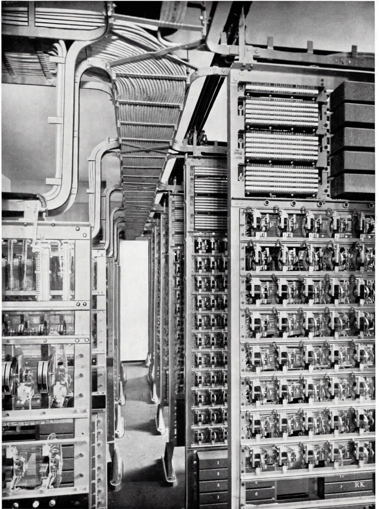
Abb. 4. SA-Eisensprechzentrale, Vereinigte Stahlwerke Düsseldorf
