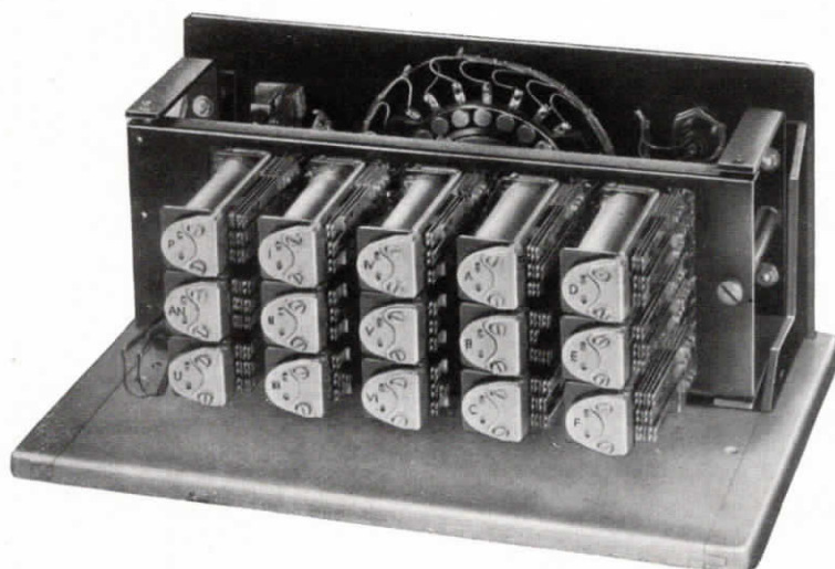
Abb. 4 Abzählgerät Innenansicht
