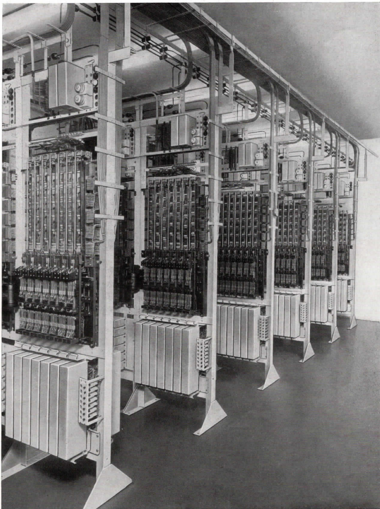
Abb. 4 Wählerraum der Rekord-Zentrale III S für 50 Amtsleitungen und 600 Nebenstellen im Büro-Hochhaus Frankfurt a. M.-Süd
