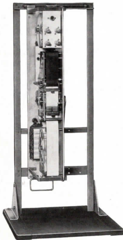
Abb. 4 Automatischer Gesprächs-zetteldrucker
