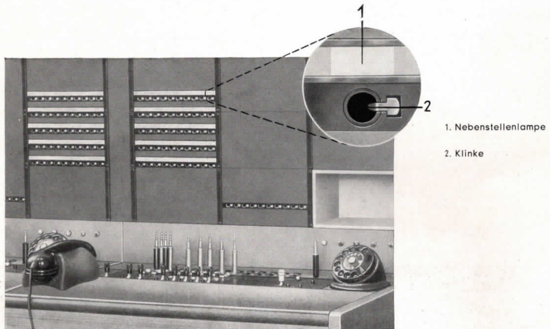
Abb. 5 Die zweifache Aufgabe der Nebenstellenlampe
