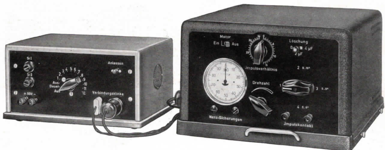
Abb. 1 Stromstoßsender mit Abzählgerät
