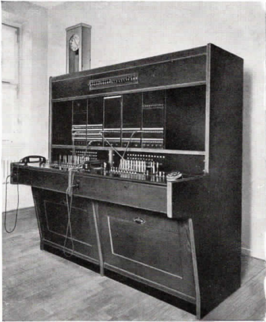
Abb. 7 2plätziger Bedienungsschrank der Rekord-Zentrale III S für 20 Amtsleitungen und 200 Nebenstellen im Arbeitsamt Frankfurt a. M.
