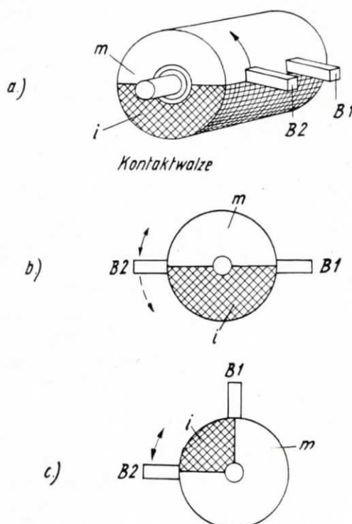
Abb. 5 Unterteilung des Kollektors
