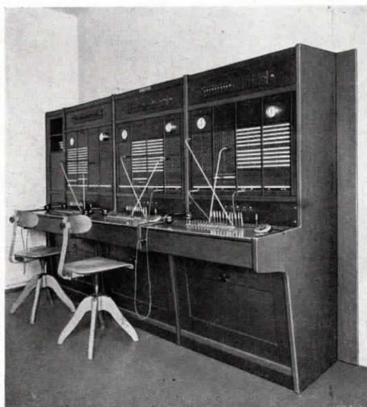
Abb. 3 3plätziger Bedienungsschrank der Rekord-Zentrale III S für 50 Amtsleitungen und 600 Nebenstellen im Büro-Hochhaus Frankfurt a. M.-Süd
