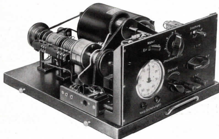
Abb. 3 Stromstoßsender Innenansicht
