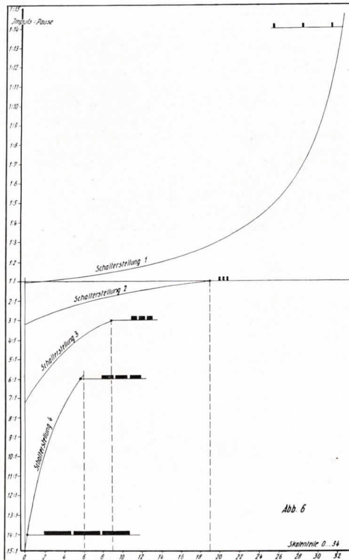
Abb. 6 Eichkurve des Stromstoßsenders
