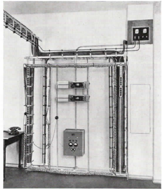
Abb. 9 Wandverteiler mit Ruf- u. Signalmaschinen u. Dauerladegerät im Arbeitsamt Frankfurt a. M.
