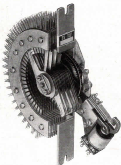
Abb. 5 Anrufsucher
