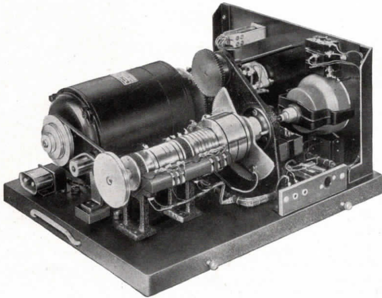
Abb. 2 Stromstoßsender Innenansicht
