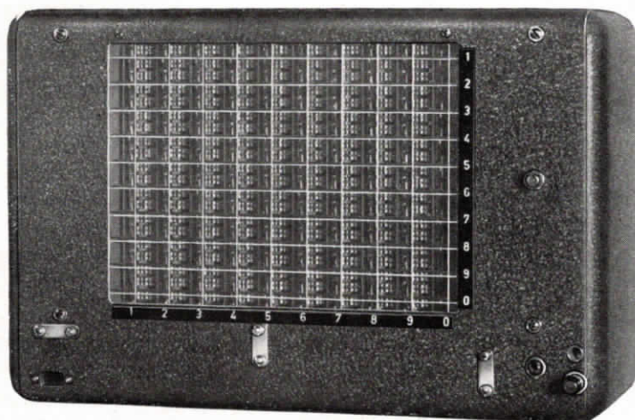
Abb. 7 100tlg. 4driger Edelmetallkontaktwähler (Kreuzschienenwähler) Gesamtansicht mit Schutzkappe
