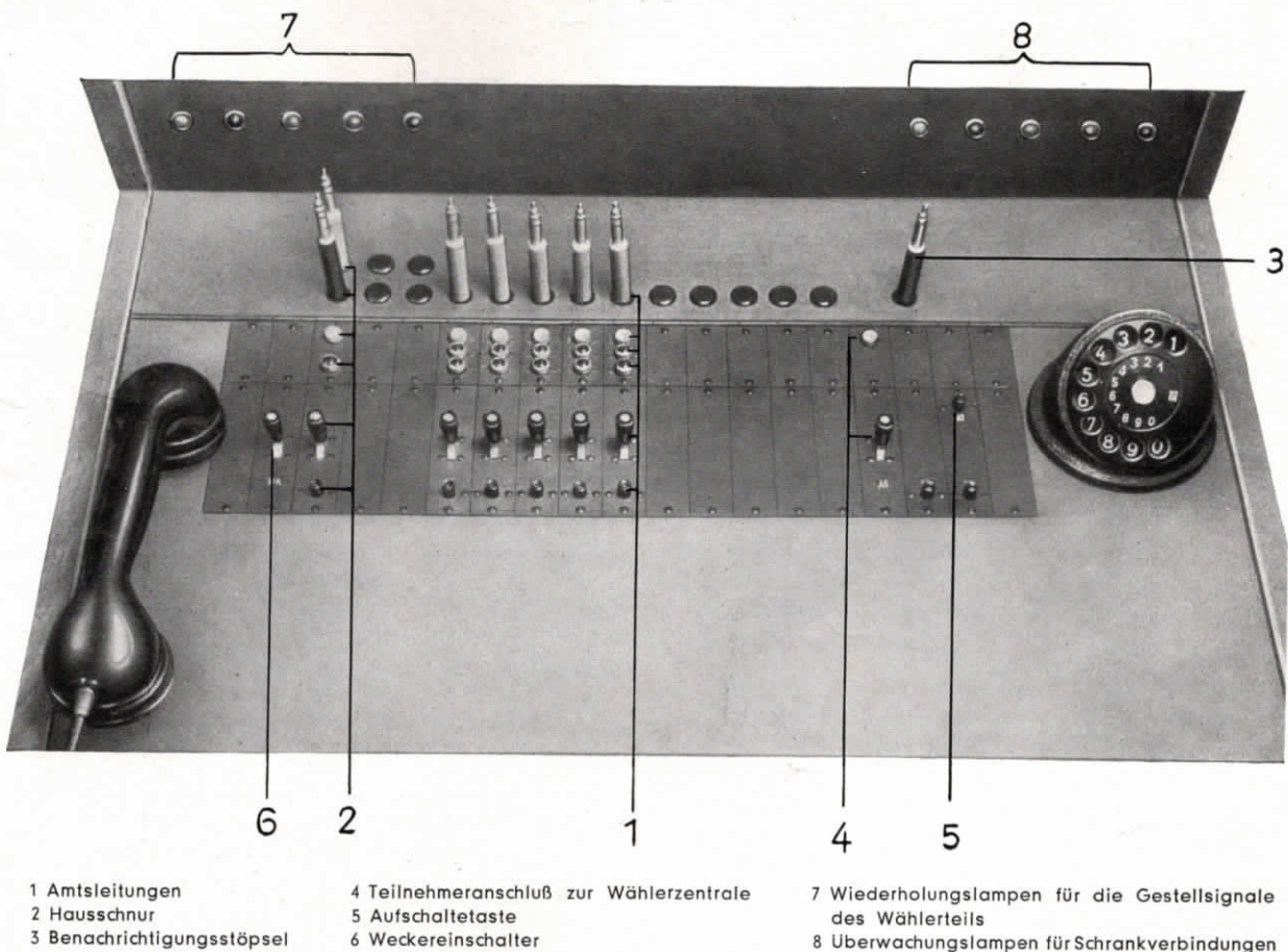
Abb. 6 Abfrage- und Bedienungsplatz einer REKORD-Zentrale (Einschnursystem)
