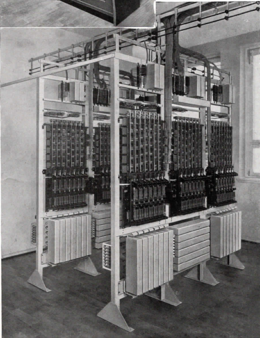
Abb. 8 Wählerraum der Rekord-Zentrale III S für 20 Amtsleitungen und 200 Nebenstellen im Arbeitsamt Frankfurt a. M.
