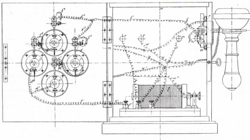
Abb. 119 Maiche-Apparat, aufgeklappt (1881)
