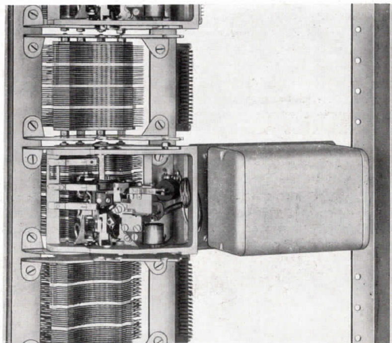
Abb. 8 Rahmenmäßiger Zusammenbau der vierarmigen Hebdrehwähler
