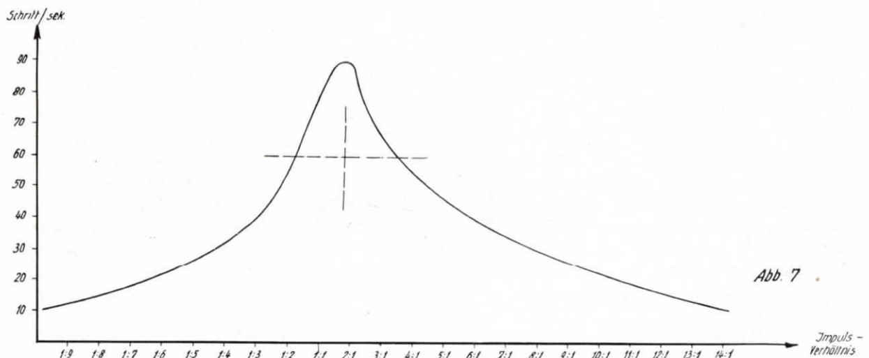
Abb. 7 Untersuchung eines 12tlg. Drehwählers
