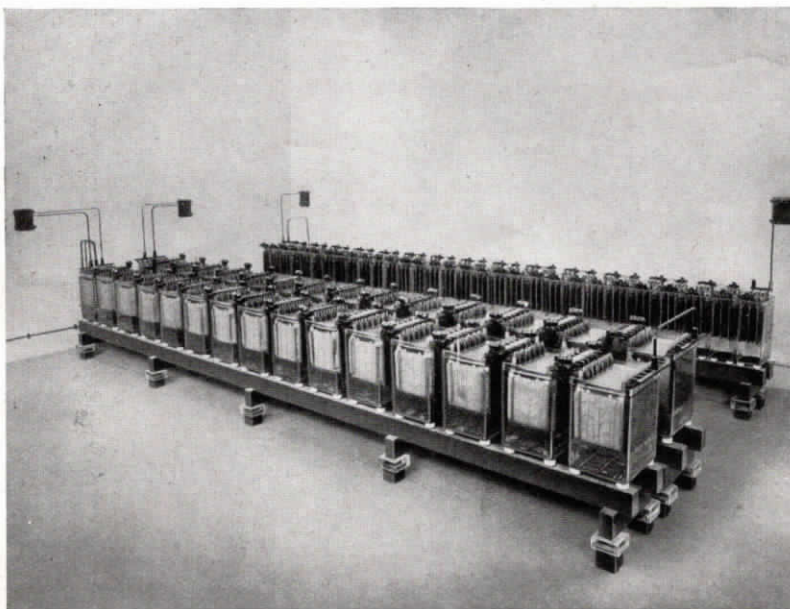
Abb. 6 Batterieraum
