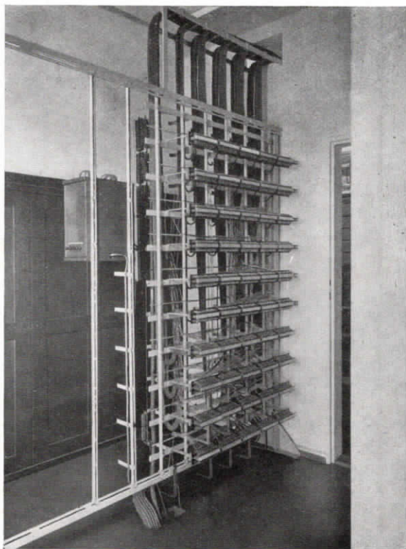
Abb. 5 Haupt- und Rangierverteiler
