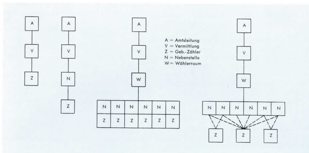
BILD 4 Schematische Übersicht des Einsatzes von Gebührenzähleinrichtungen
