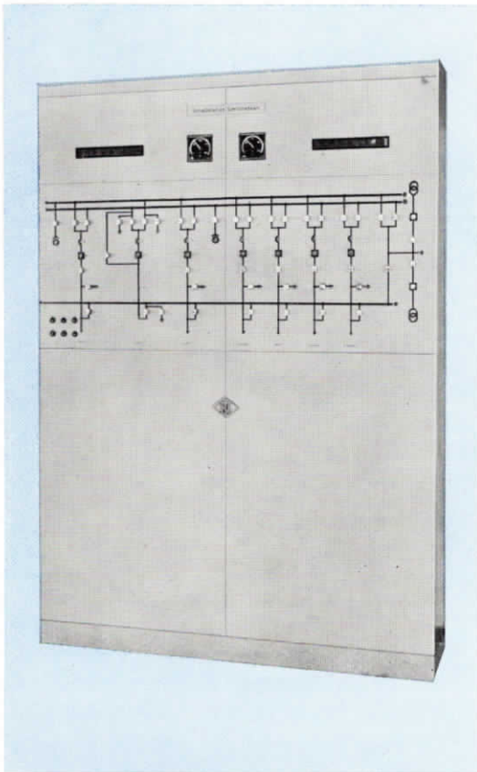
BILD 13 Bedienungstafel der Leitstelle Kirchhain
