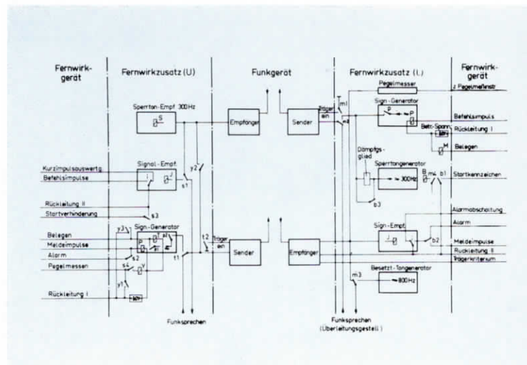
BILD 5 Grundsaltbild der Fernwirkzusätze
