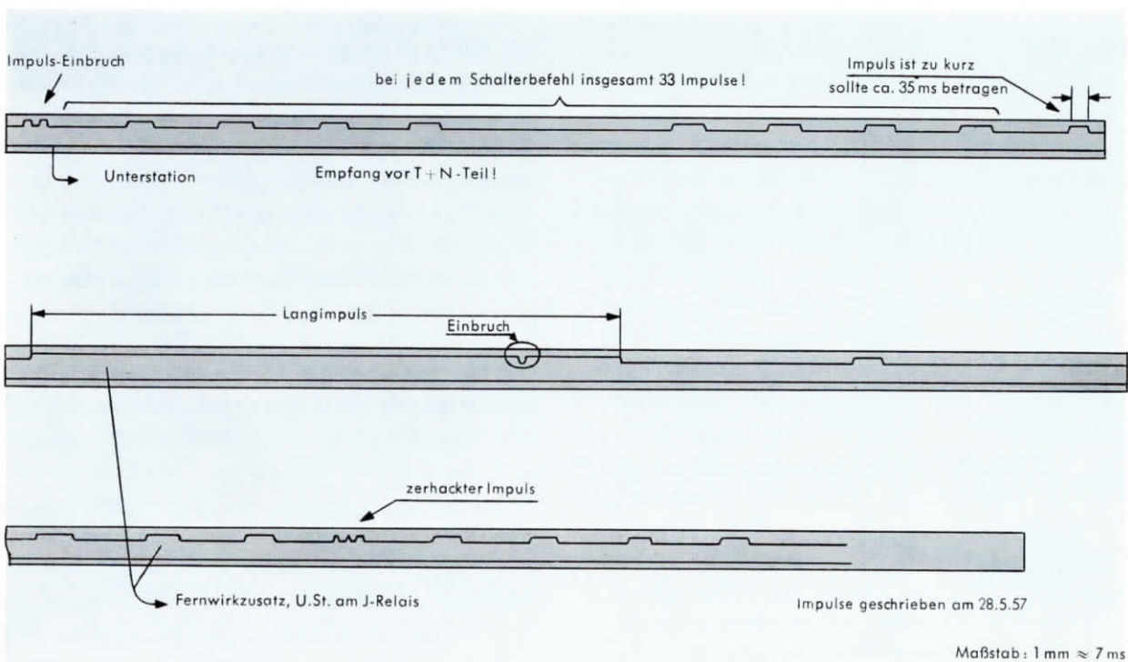
BILD 15 Impulstelegramm von Kommando- zur Unterstation
