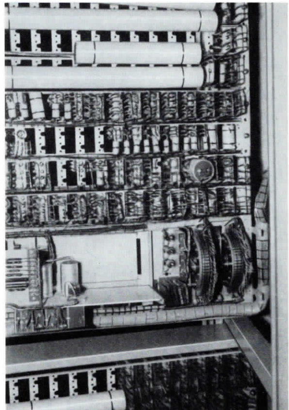
BILD 14 Relaisteil des Fernwirkgerätes der Leitstelle
