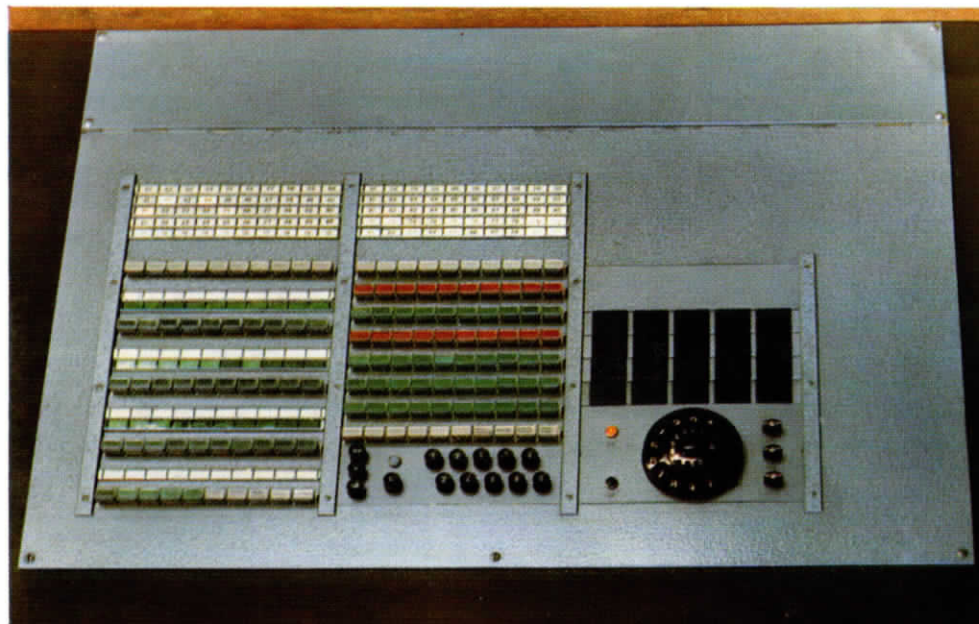
Bedienungsfeld des Aufsichtsplatzes
