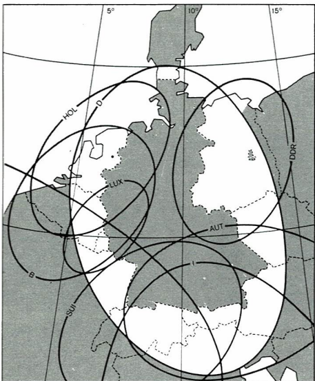
Die Bedeckungsgebiete der Rundfunk-Satelliten für die Position 19° W (Mitteleuropa)
