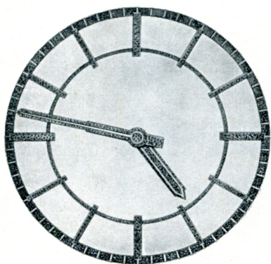
Nr. 431 98/31 Ringe, Zeiger und Stundenstriche aus gehämmertem Schmiedeeisen, Minutenstriche aus Messing 30, 40, 50, 60, 80 und 100 cm \phi
