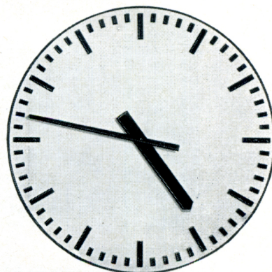
Nr. 431 98/13 Elfenbeinfarbiges Zifferblatt; Zeiger, Ring und Striche aus brüniertem Messing 30, 40, 50, 60, 80 und 100 cm \phi
