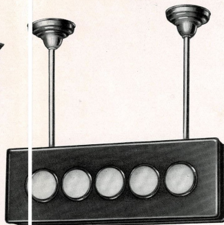
Freihängendes Tablo, doppel- seitig leuchtend, für Ruf- und Suchzwecke
