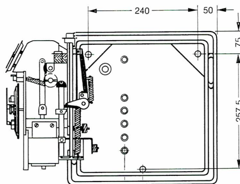
Maße in mm Gewicht ca. 21,5 kg netto
